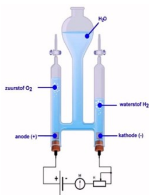
Laboratorium module om waterstof te genereren.
